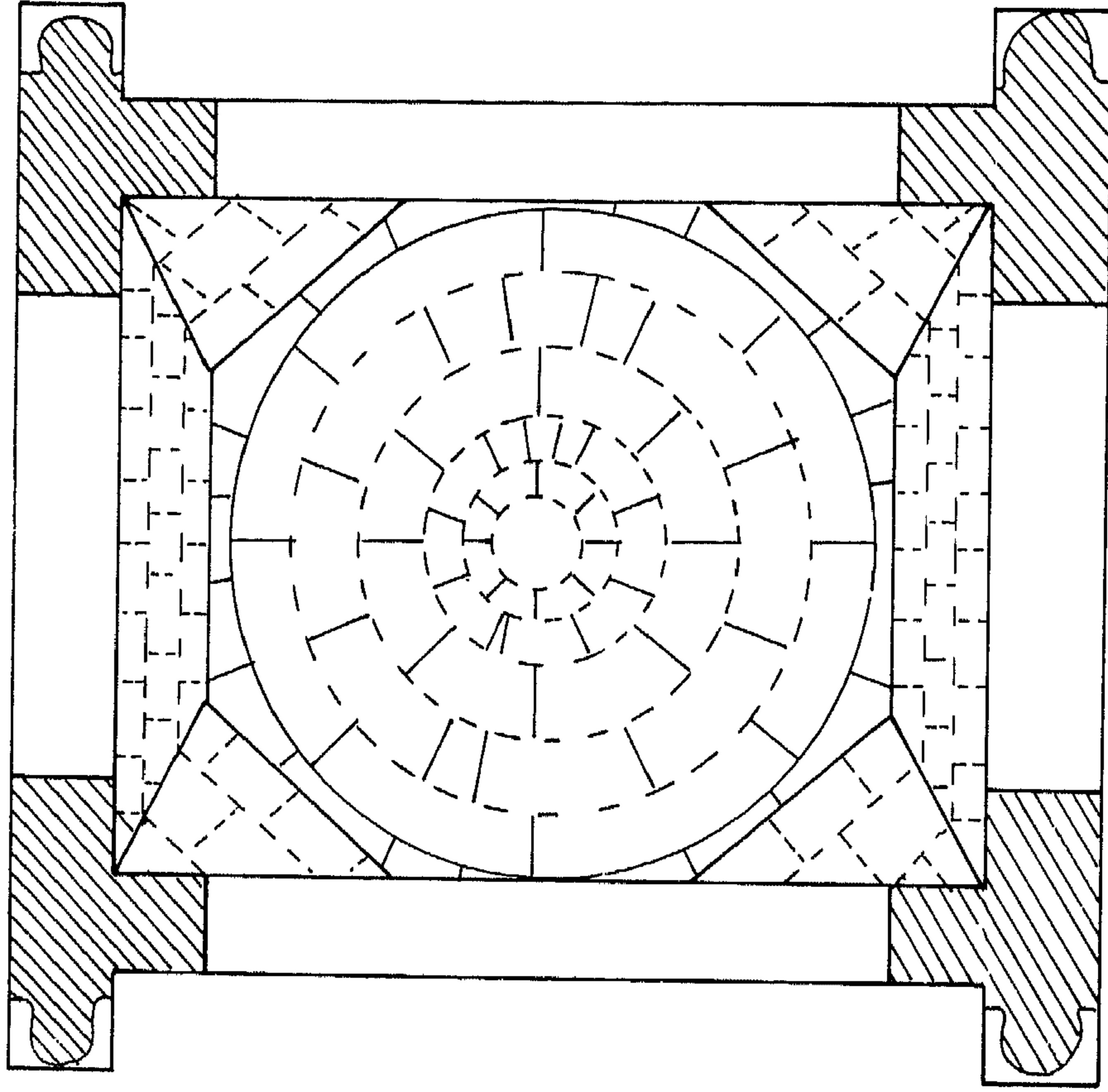
شكل (٢٤) مخطط التيترايبلون في اللاذقية (عن : Creswell, Fig.368)
